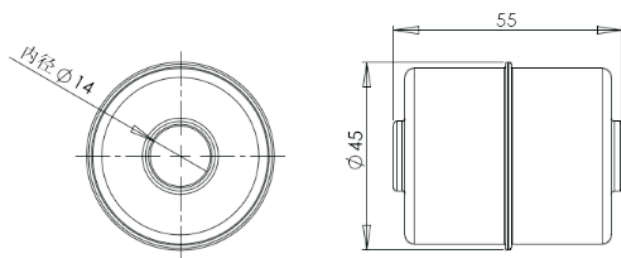
带显示磁性浮球外形尺寸图
